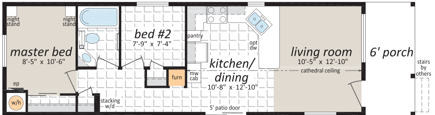
“The Riverview” 14' x 50', 616 sq. ft., 2FL-1B
